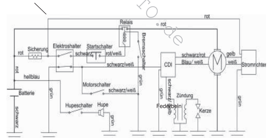
SCHALTPLAN-KXD609:
